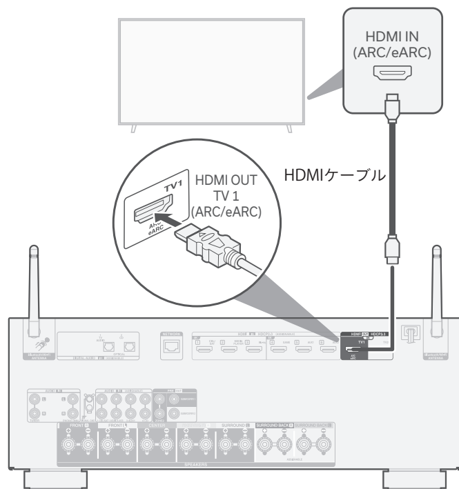
本機（リアパネル）
